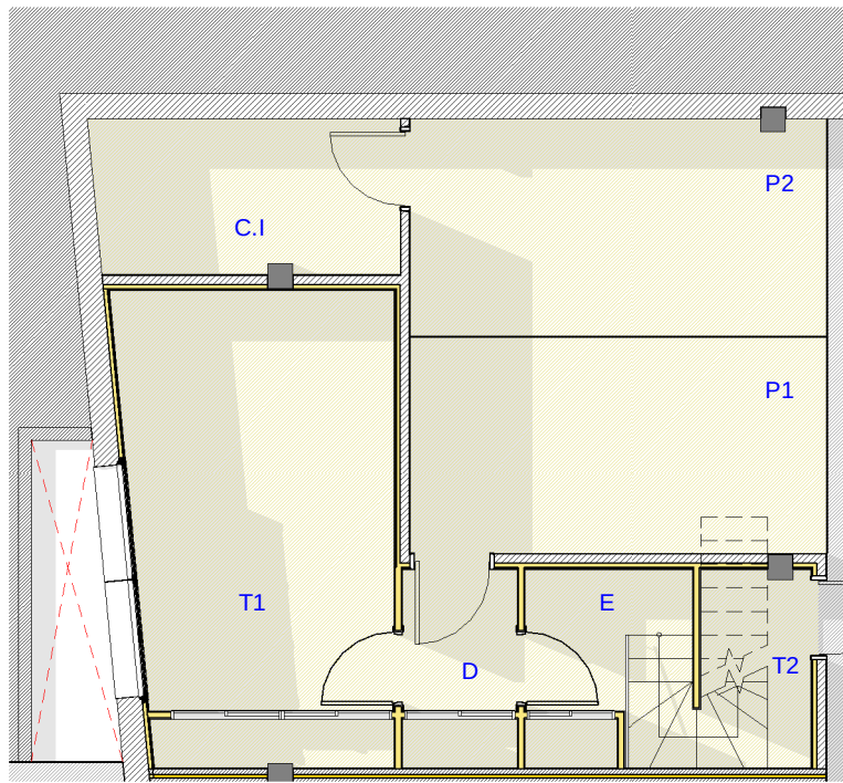
② VIV. 16C - P.S. 1 : 100
