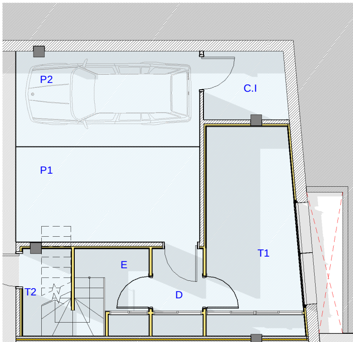
② VIV. 16B - P.S. 1 : 100
