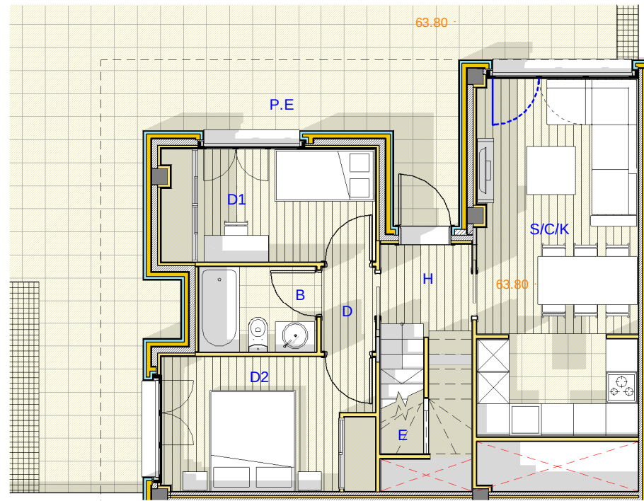
③ VIV. 16C - P.B. 1 : 100
