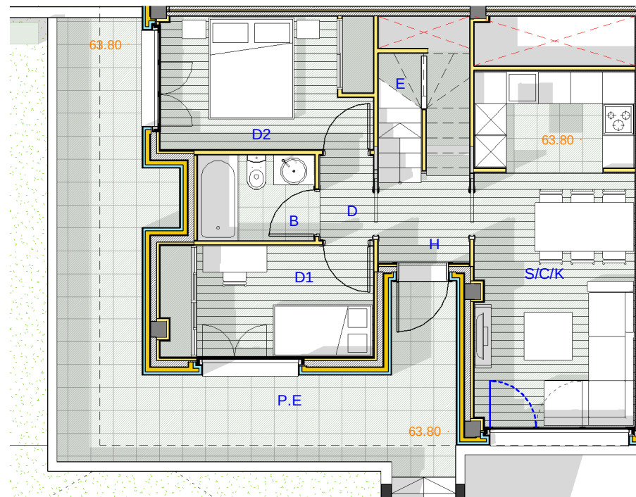
③ VIV. 16A - P.B. 1 : 100
