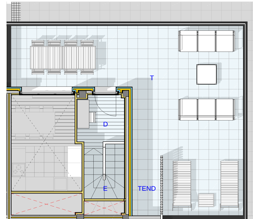
④ VIV. 16B - P.A. 1 : 100
