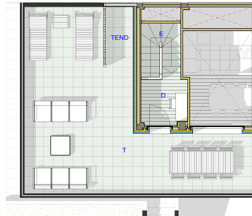
④ VIV. 16A - P.A. 1 : 100
