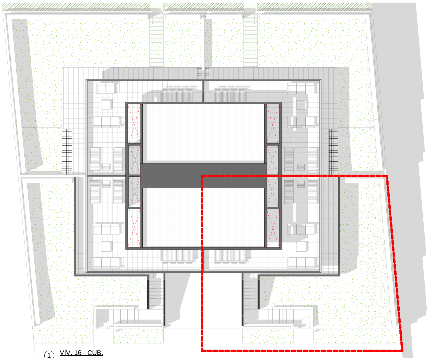
① VIV. 16 - CUB. 1 : 200
