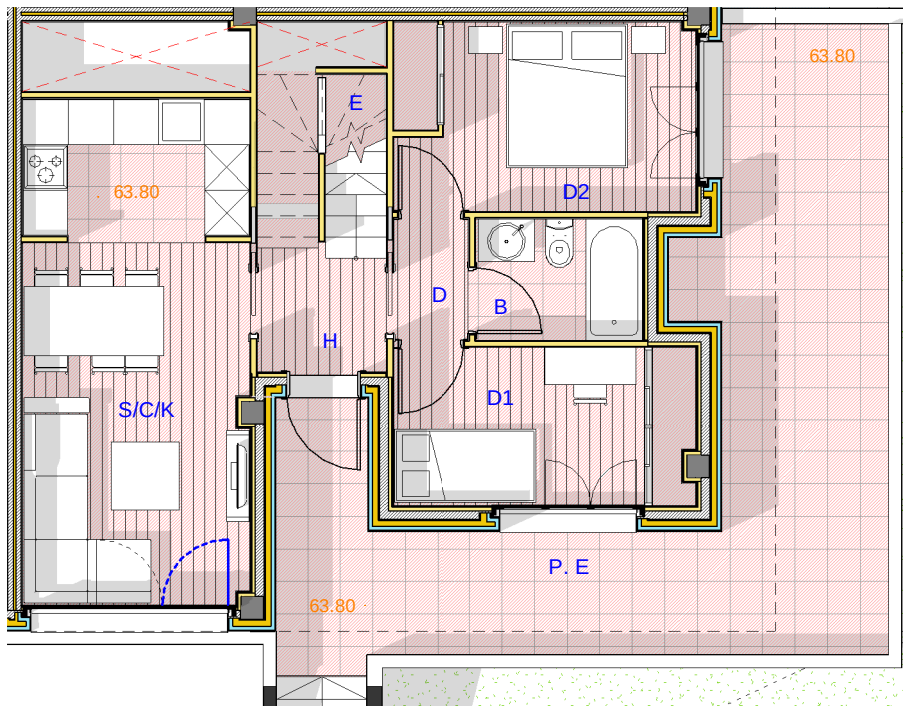
③ VIV. 16 - P.B. 1 : 100
