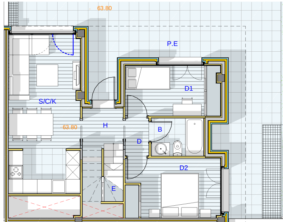
③ VIV. 16B - P.B. 1 : 100
