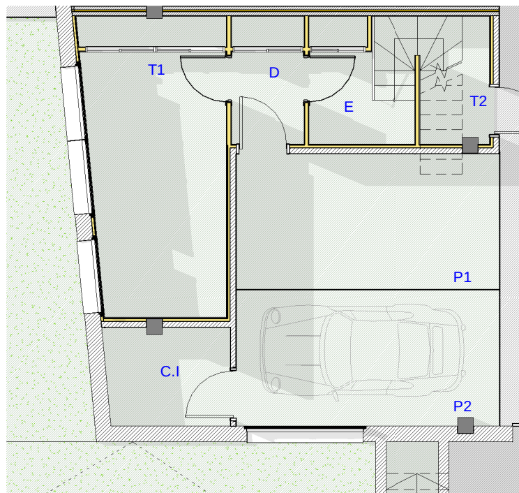
② VIV. 16A - P.S. 1 : 100
